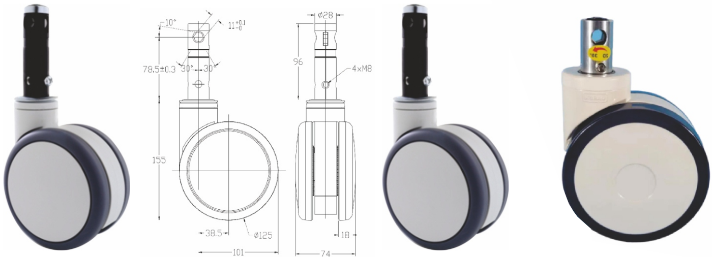
IV62-TW-CLC-3N/30- 125 -D28X96
